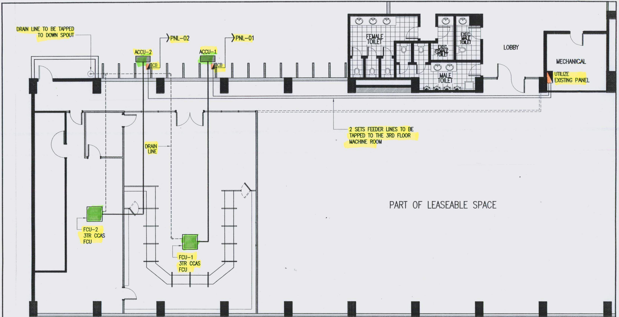
1 A/C LAYOUT SCALE: A3-1:100M/A4-1:150M
